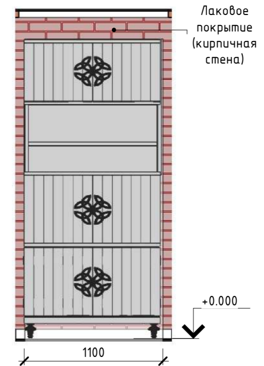
Развертка 65 -3 М 1: 30
