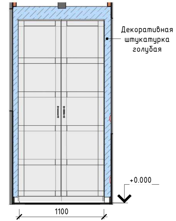
Развертка 66 -2 М 1 : 30
