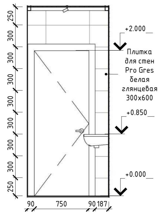
Развертка 63 -4 М 1: 30
