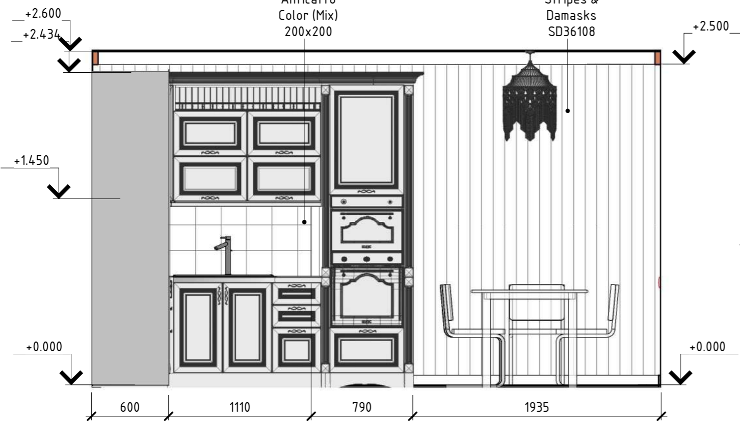
Развертка 62 -1
