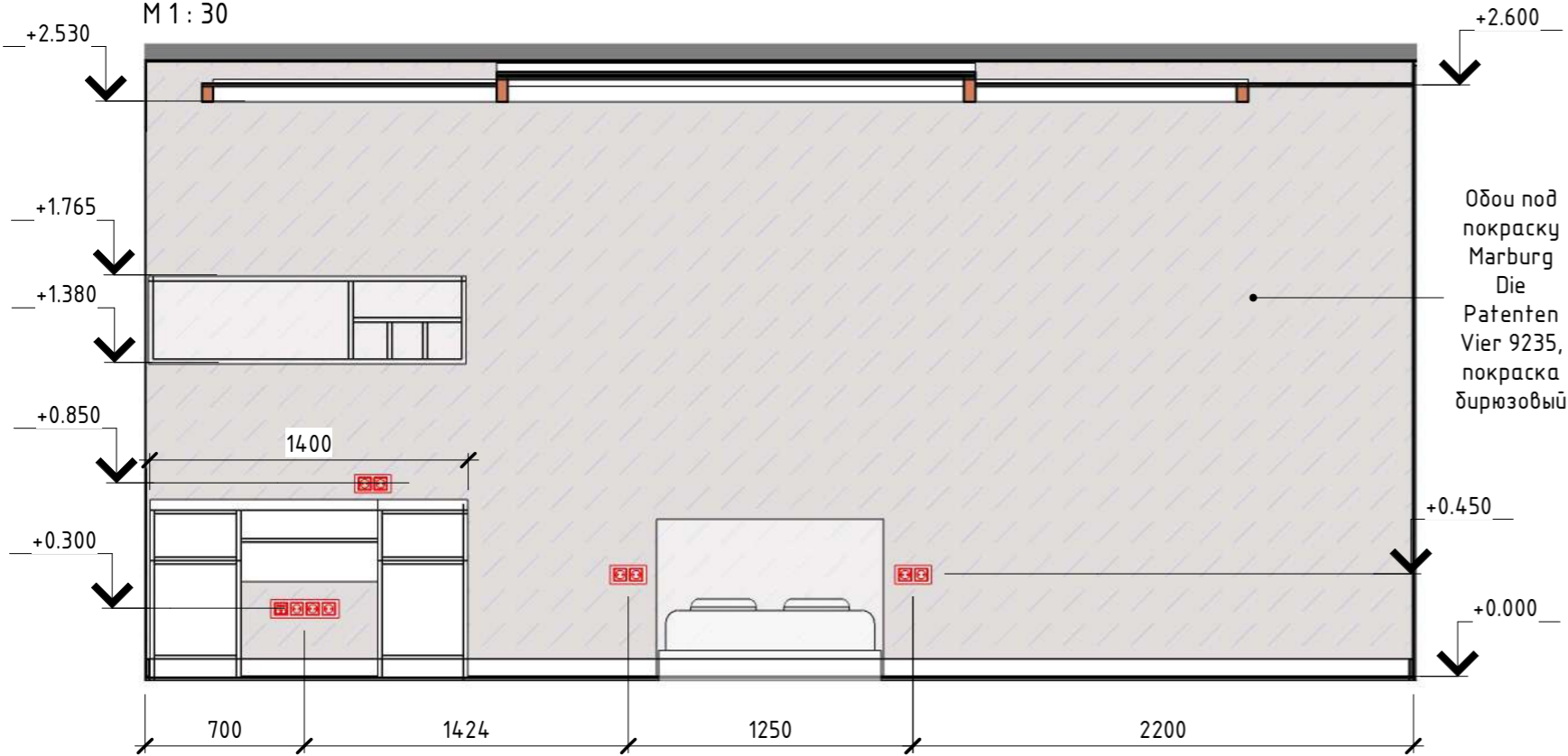
Развертка 56 -1 М 1 : 30
