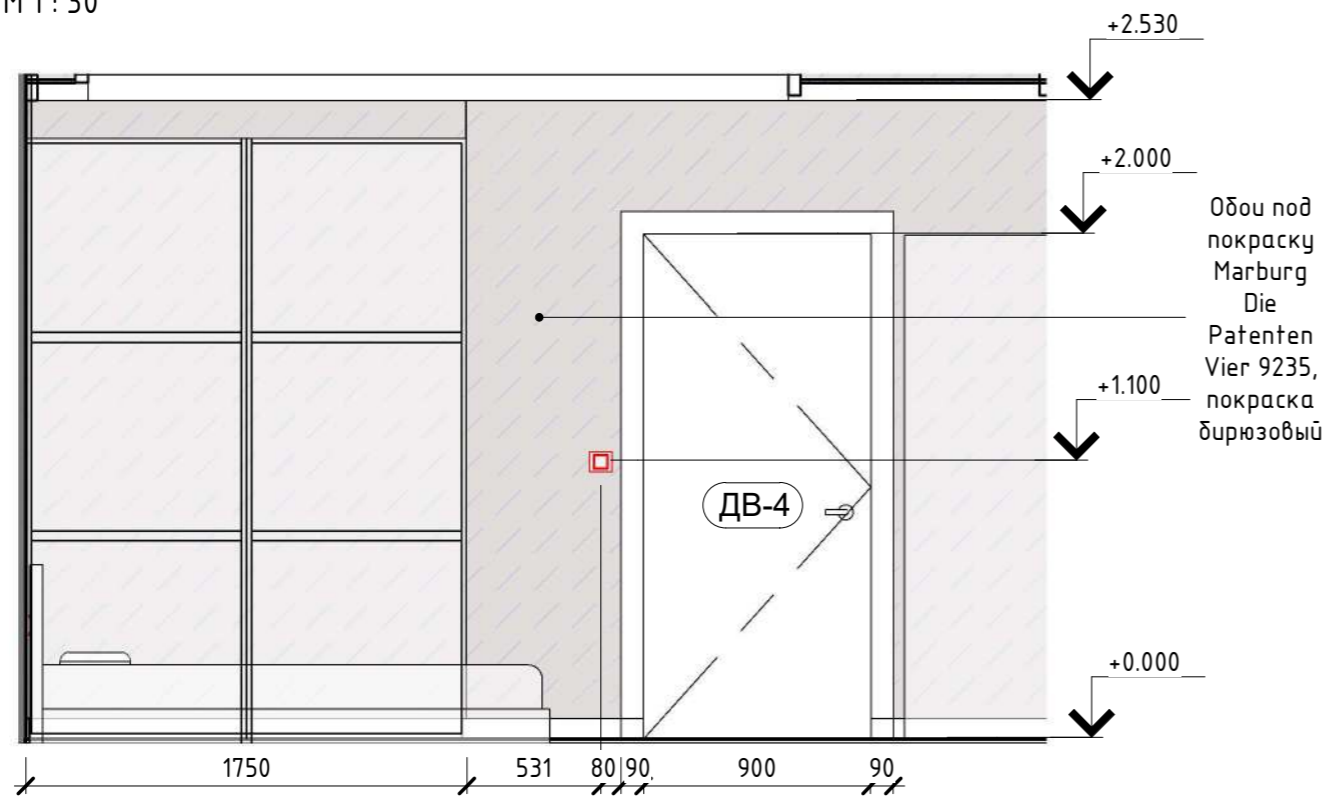
Развертка 56 -2 М 1 : 30
