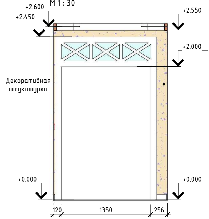
Развертка 55 -2 М 1 : 30
