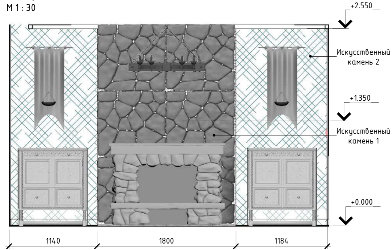
59-1 (копия 1) 1: 30
