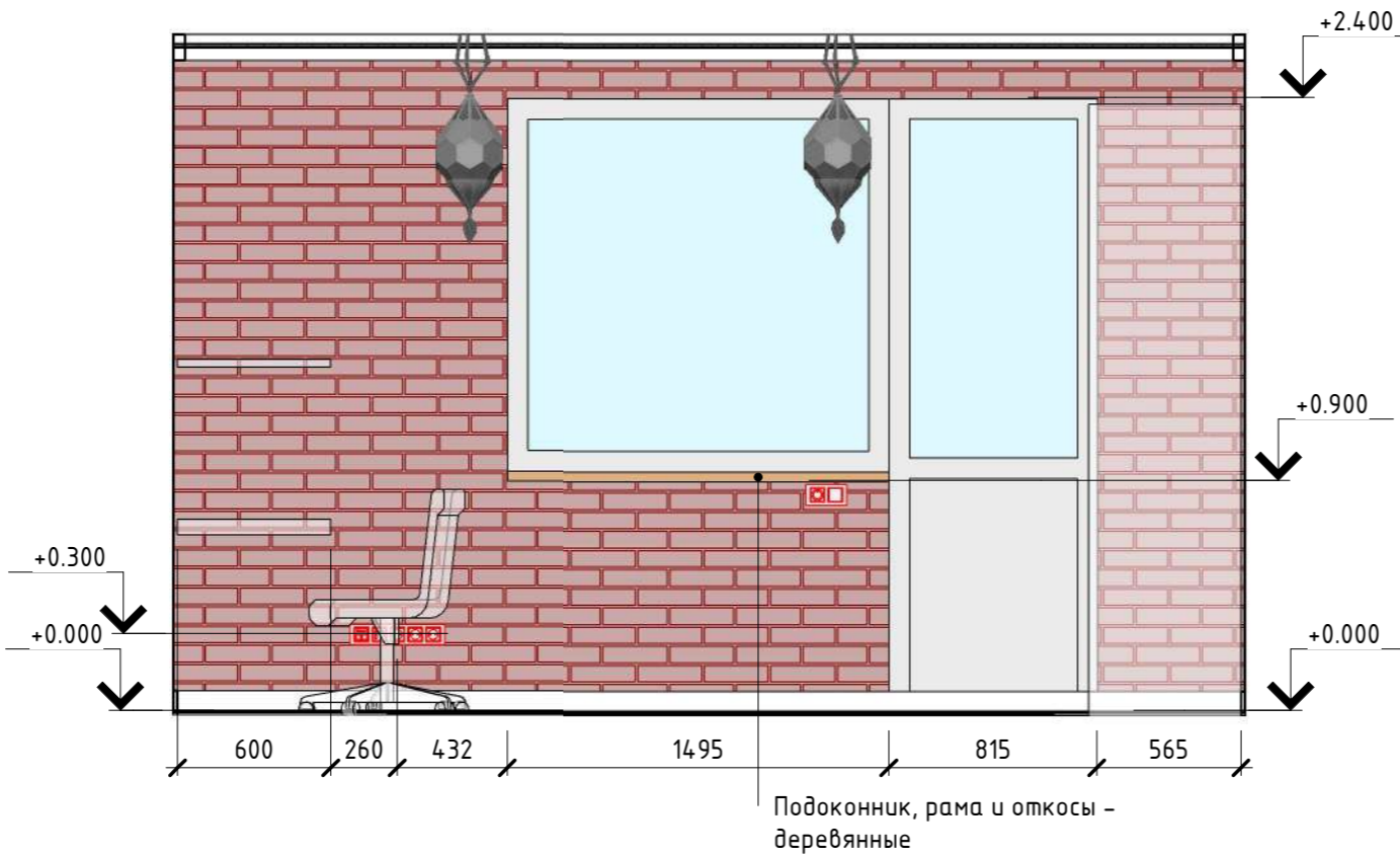
Развертка 65 -2 М 1: 30
