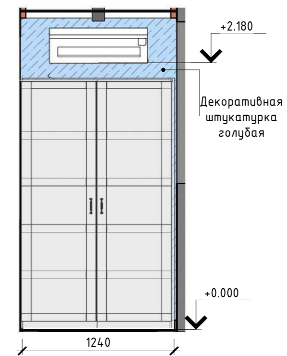
Развертка 66 -4 М 1 : 30
