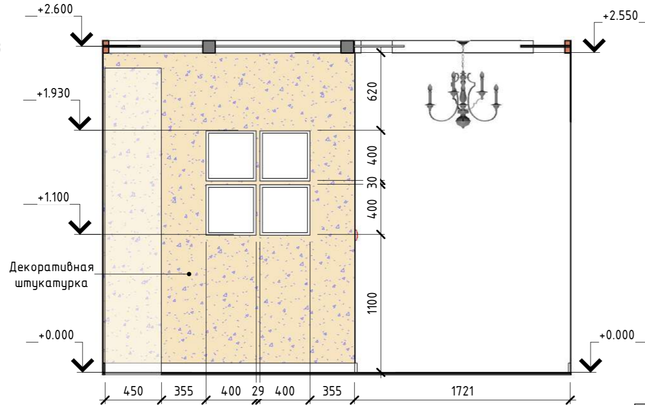
Развертка 54 -3 М 1: 30
