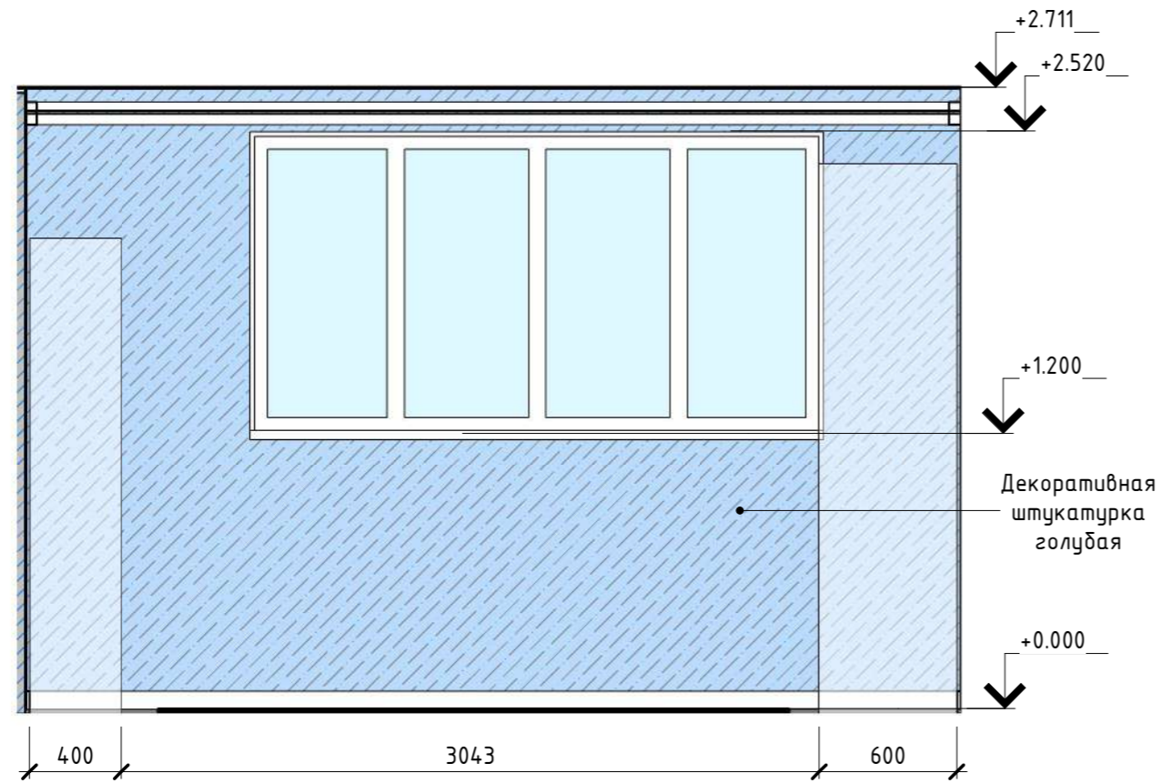
Развертка 66 -1 М 1 : 30
