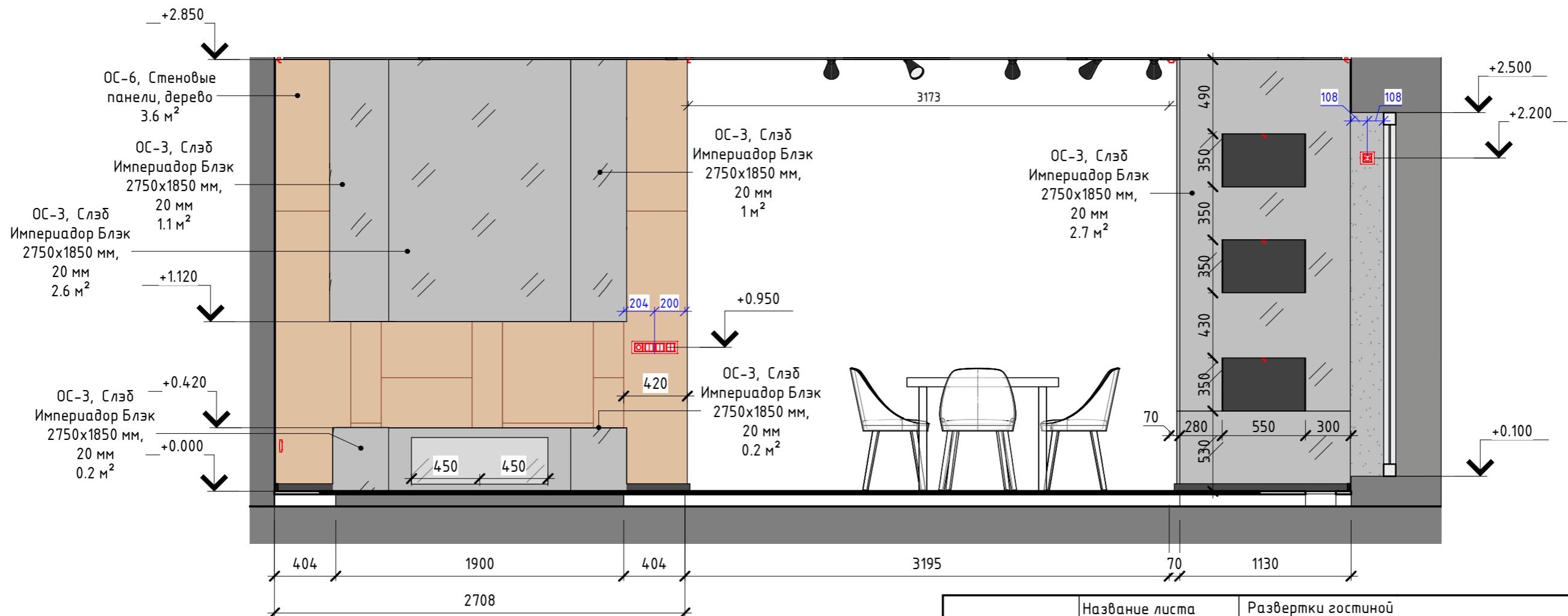
Развертка 64-2 1:30
