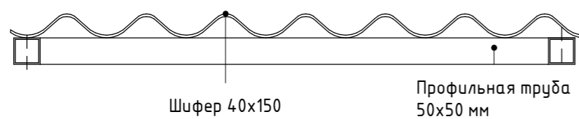
Сечение навеса над мангалом, М 1:10
