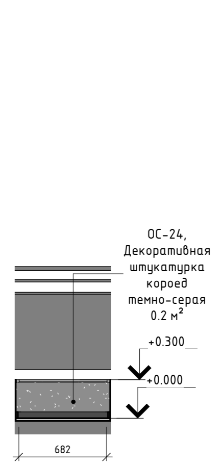
Развертка 100-3 1:30
