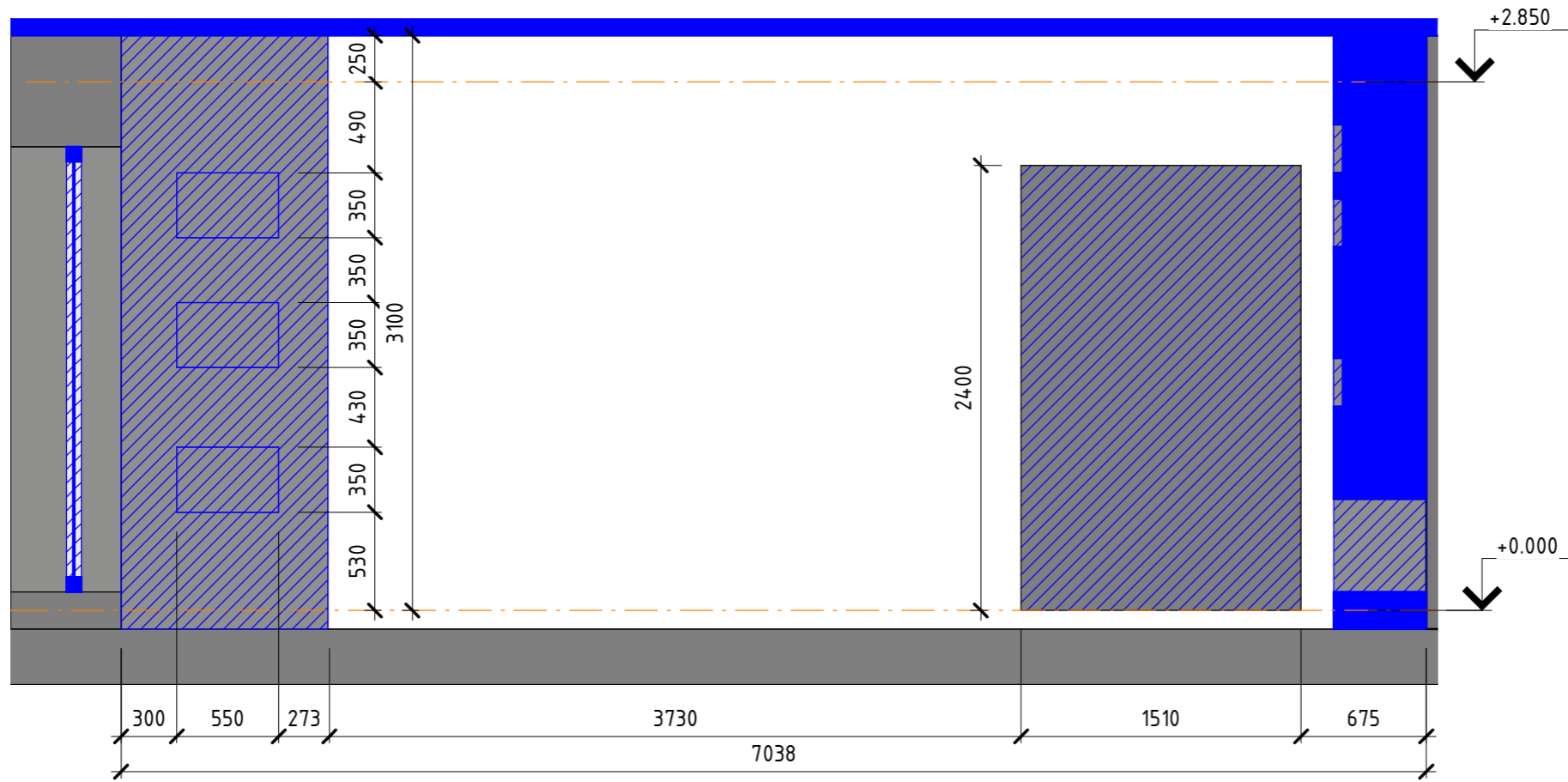
Развертка 12-1 1:35
