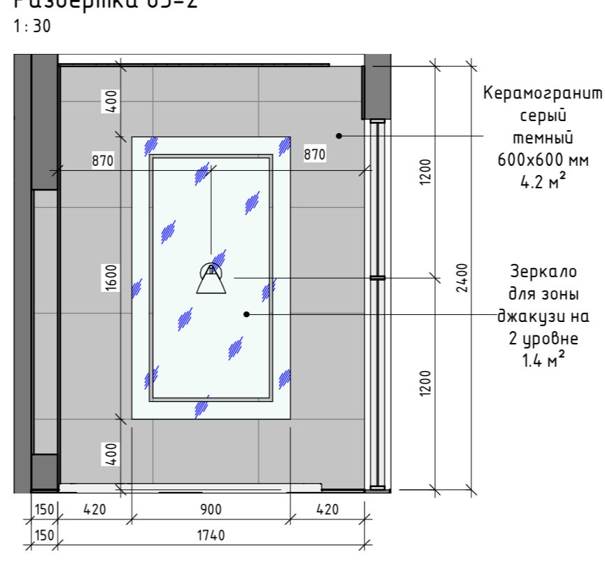
Развертка 83-2
