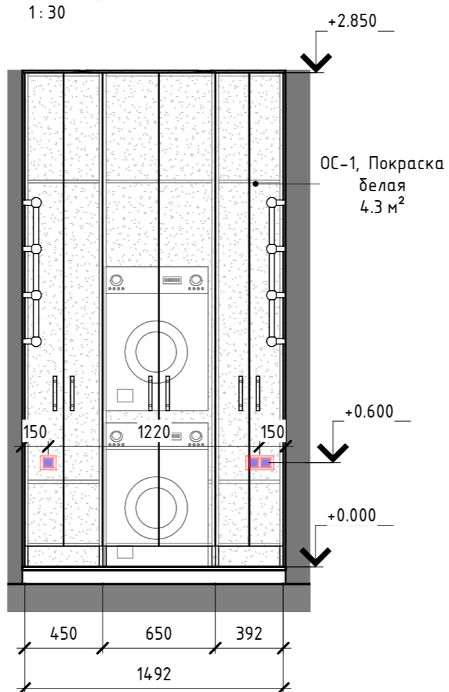
Развертка 61-2
