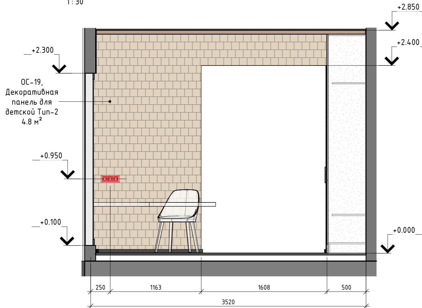
Развертка 72-3 1:30
