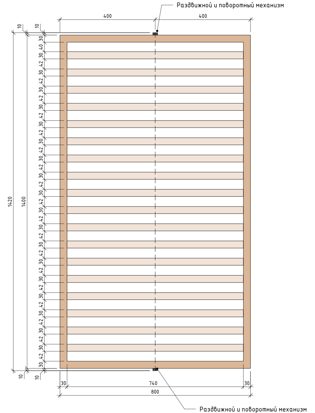
Панель К-4 с поворотным и раздвижным механизмом, 800x1400 мм
