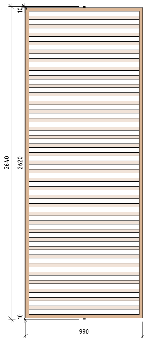
Панель К-6 с поворотным механизмом 990x2620 мм
