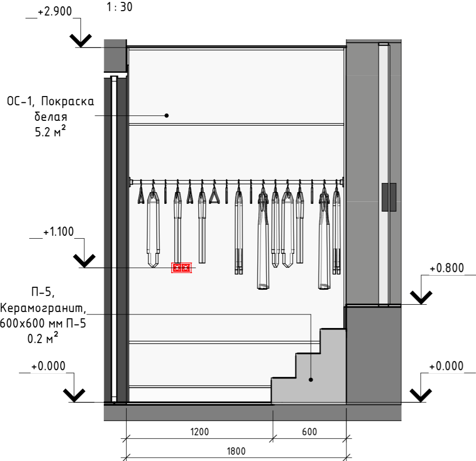
Развертка 84-1
