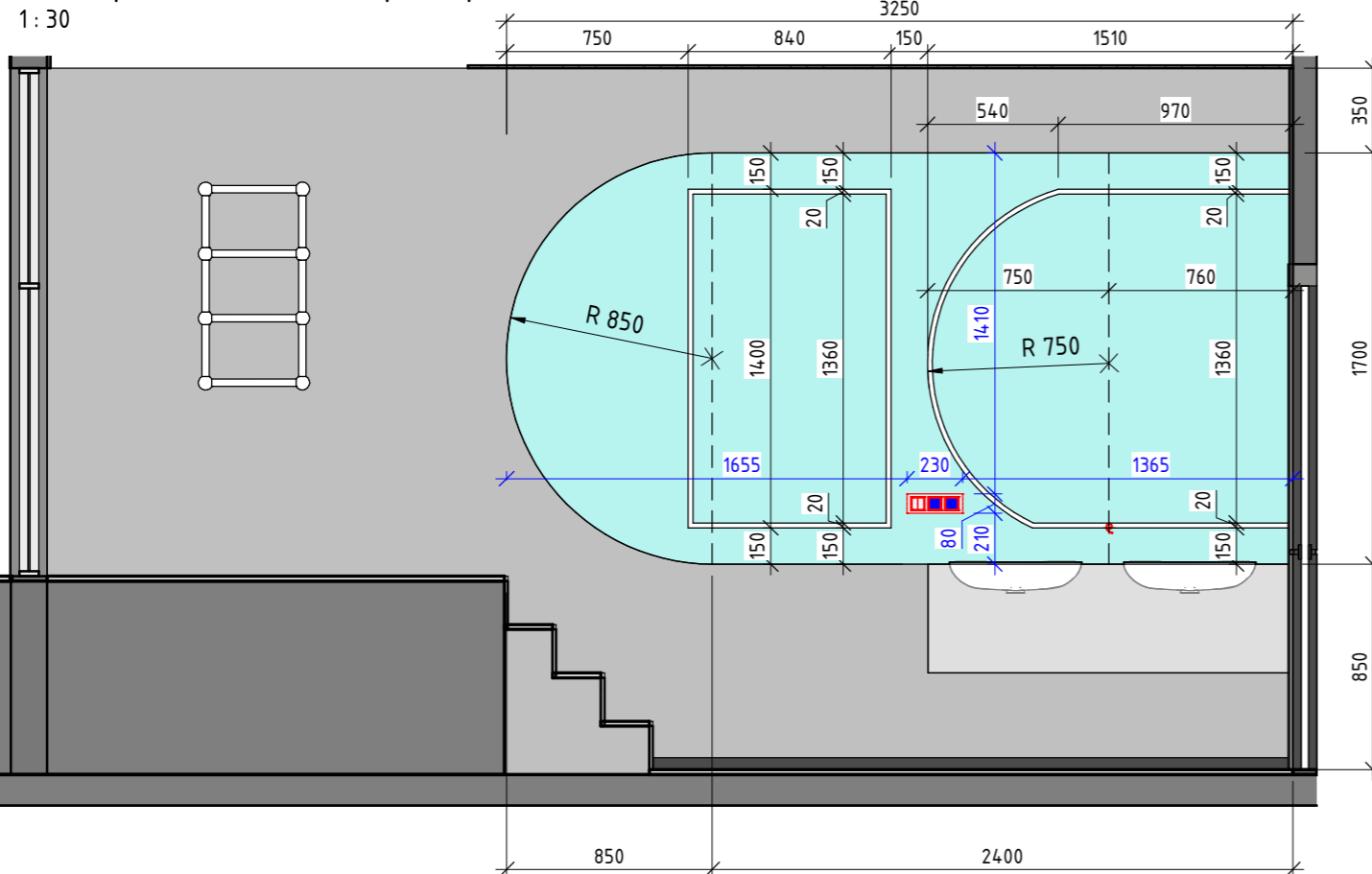
Развертка 85-1 (Размеры зеркала)
