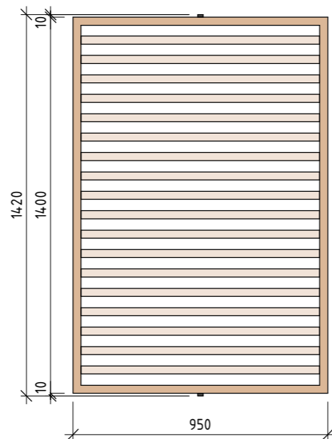
Панель К-5 с поворотным и раздвижным механизмом 950x1400 мм
