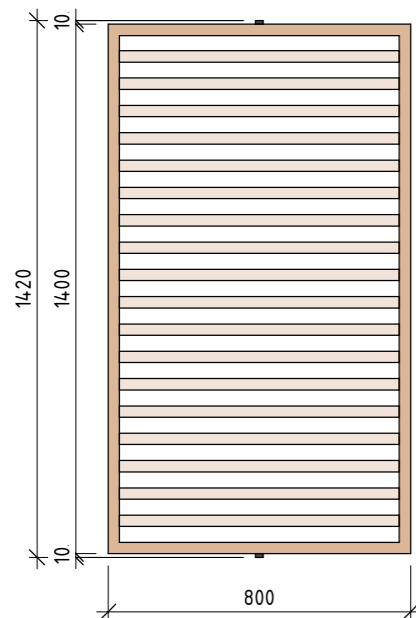
Панель К-4 с поворотным и раздвижным механизмом 800x1400 мм
